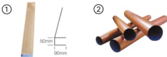
선홍통 ① 사각형 : 길이 3,000mm[90mm * 50mm] ② 원형 : 길이 900mm[65Ø or 90Ø]
